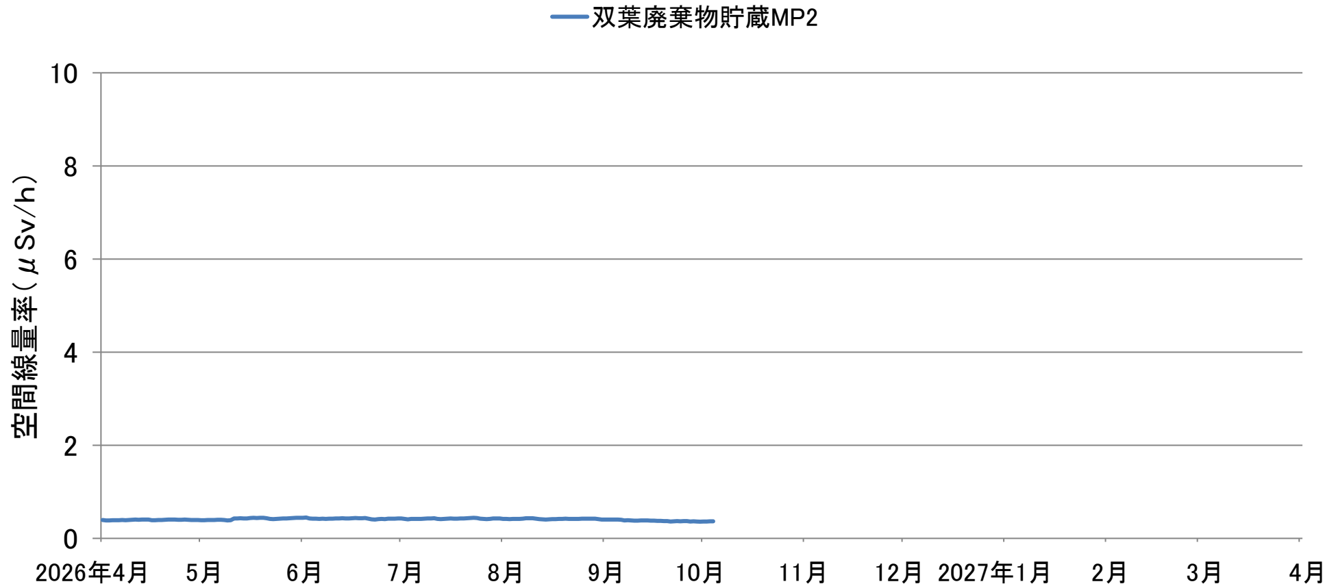
廃棄物貯蔵施設（双葉2工区）境界における空間線量率の推移（連続測定） （2026年4月1日～10月4日）
