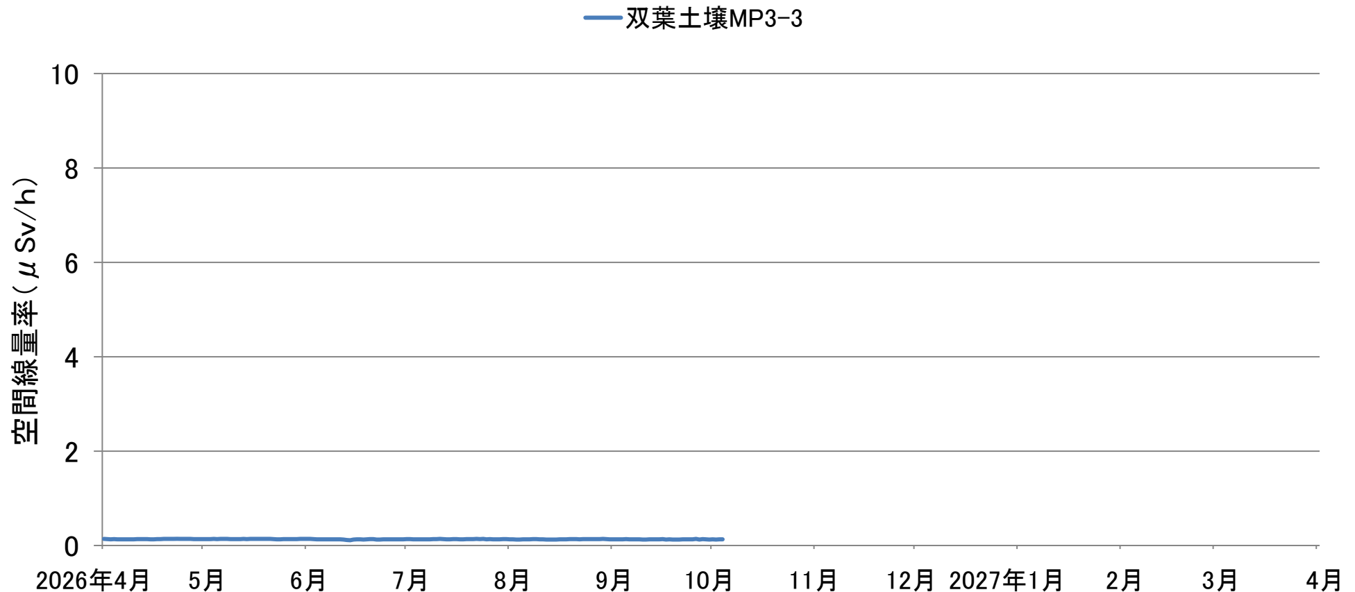
土壌貯蔵施設（双葉③工区）境界における空間線量率の推移（連続測定） （2026年4月1日～10月4日）
