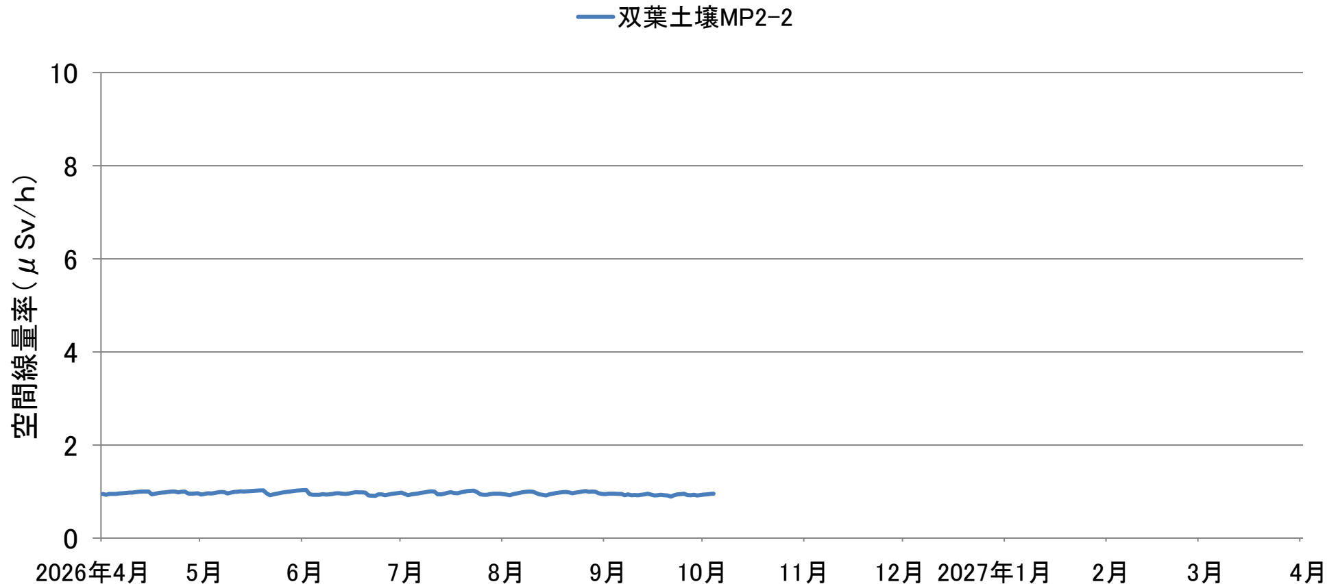
土壌貯蔵施設（双葉②工区）境界における空間線量率の推移（連続測定） （2026年4月1日～10月4日）
