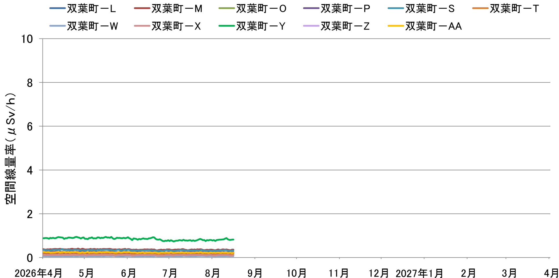
保管場等境界における空間線量率の推移(連続測定) (2026年4月1日～8月16日)
