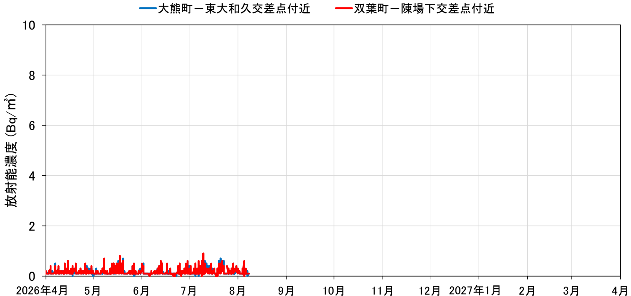
中間貯蔵施設区域境界における大気中の \beta 線の放射能濃度(連続測定) (2026年4月1日～8月7日)
