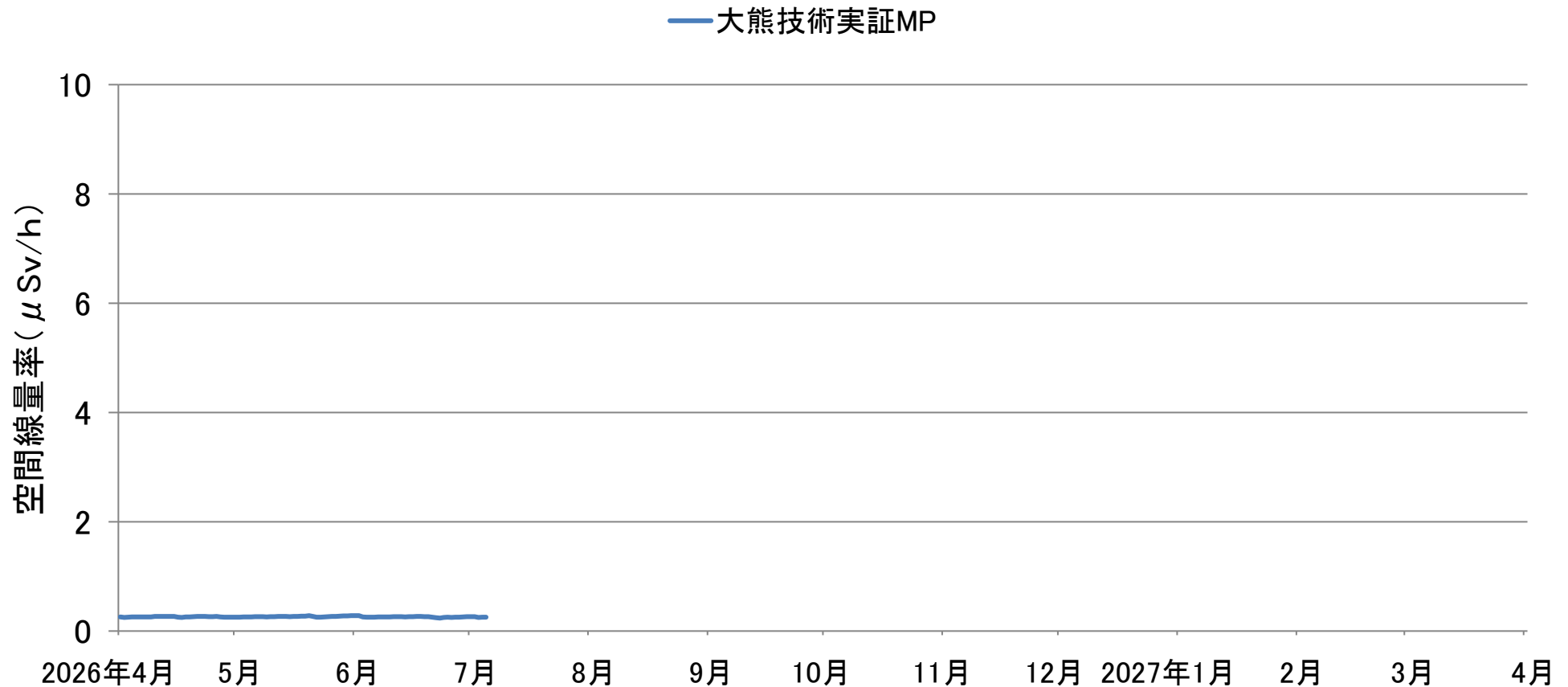
技術実証フィールド敷地内における空間線量率の推移（連続測定） （2026年4月1日～7月5日）
