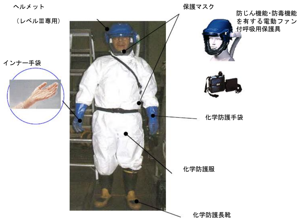
図 9-4 解体撤去管理レベルⅢの保護具の例
