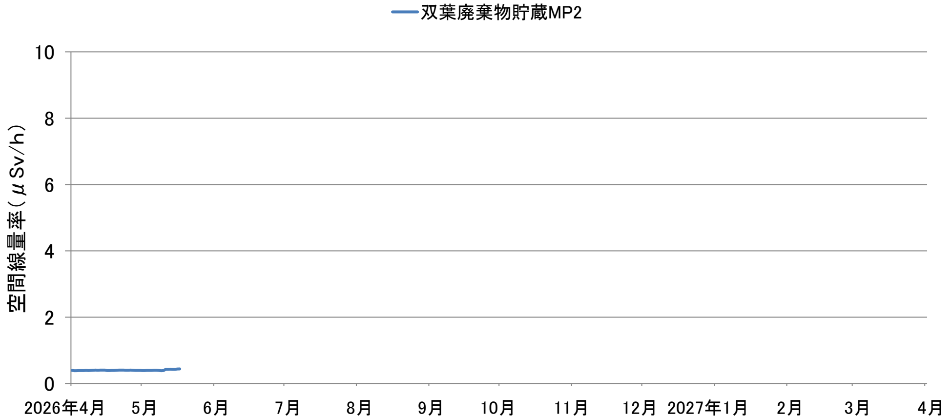
廃棄物貯蔵施設（双葉2工区）境界における空間線量率の推移（連続測定） （2026年4月1日～5月17日）
