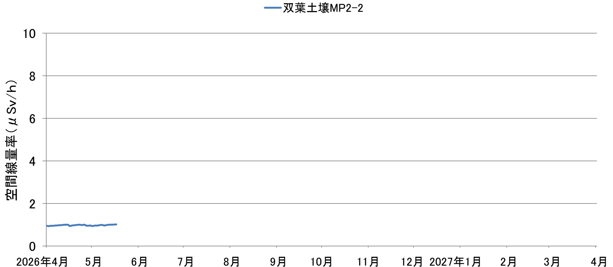
土壤貯蔵施設（双葉②工区）境界における空間線量率の推移（連続測定） （2026年4月1日～5月17日）
