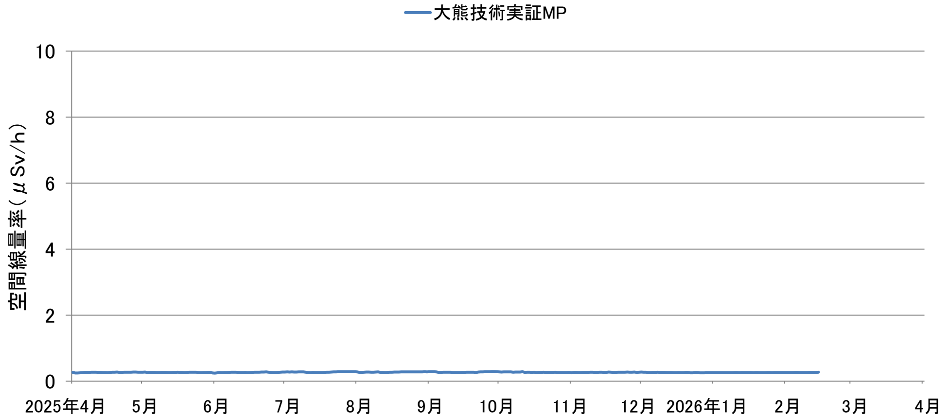
技術実証フィールド敷地内における空間線量率の推移（連続測定） （2025年4月1日 ～ 2026年2月15日）
