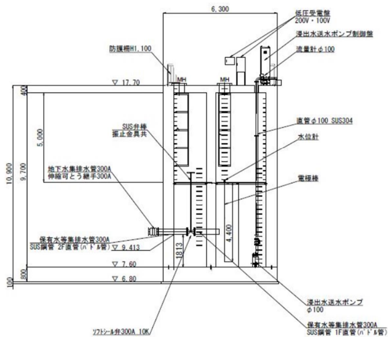
浸出水集水ピット断面図(B-B)
