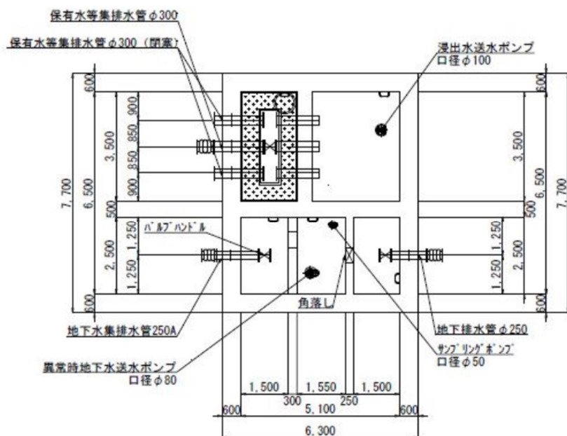
浸出水集水ピット断面図(B-B)
