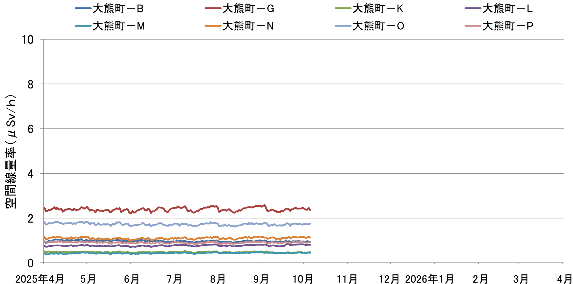
保管場等境界における空間線量率の推移(連続測定) (2025年4月1日 ~ 10月5日)
