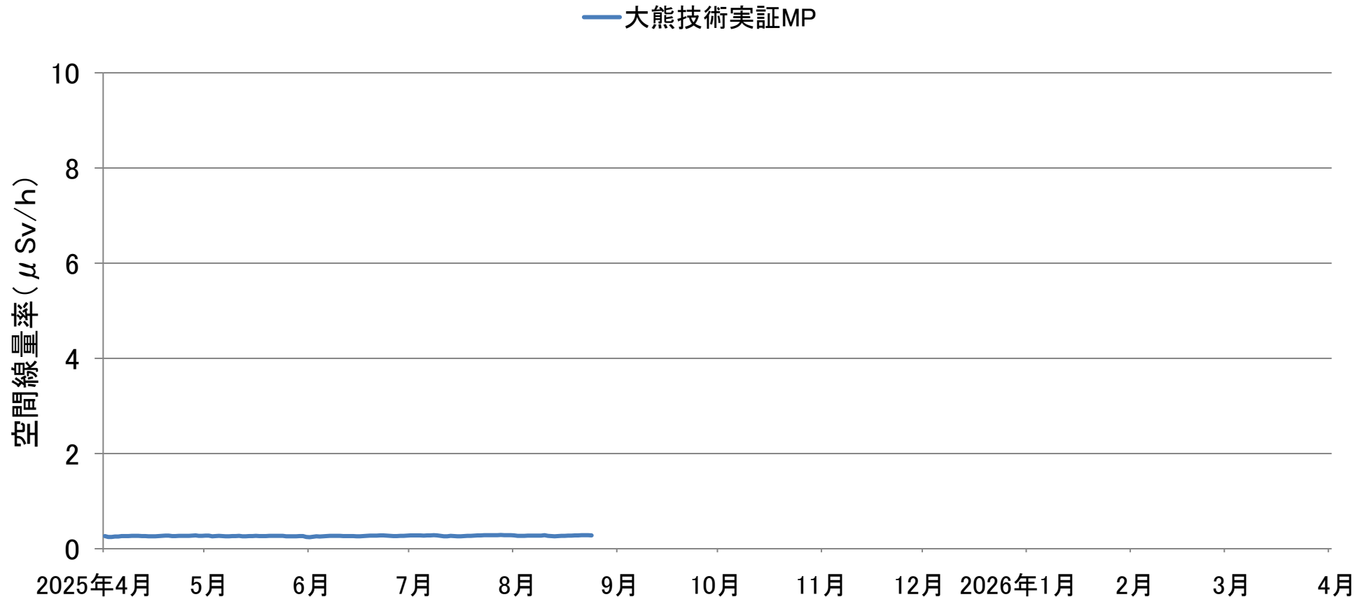
技術実証フィールド敷地内における空間線量率の推移（連続測定） （2025年4月1日～8月24日）
