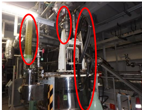
No.2遠心脱油機 配管類取り外し前
