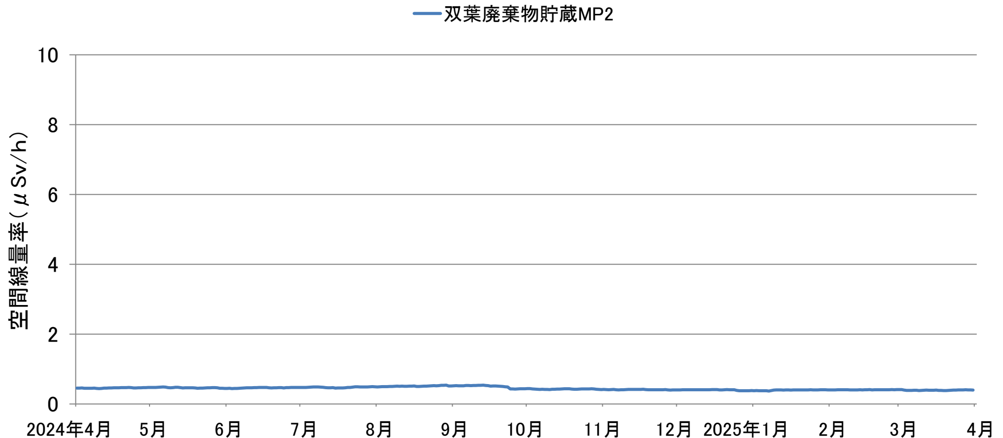
廃棄物貯蔵施設（双葉2工区）境界における空間線量率の推移（連続測定） （2024年4月1日～2025年3月31日）
