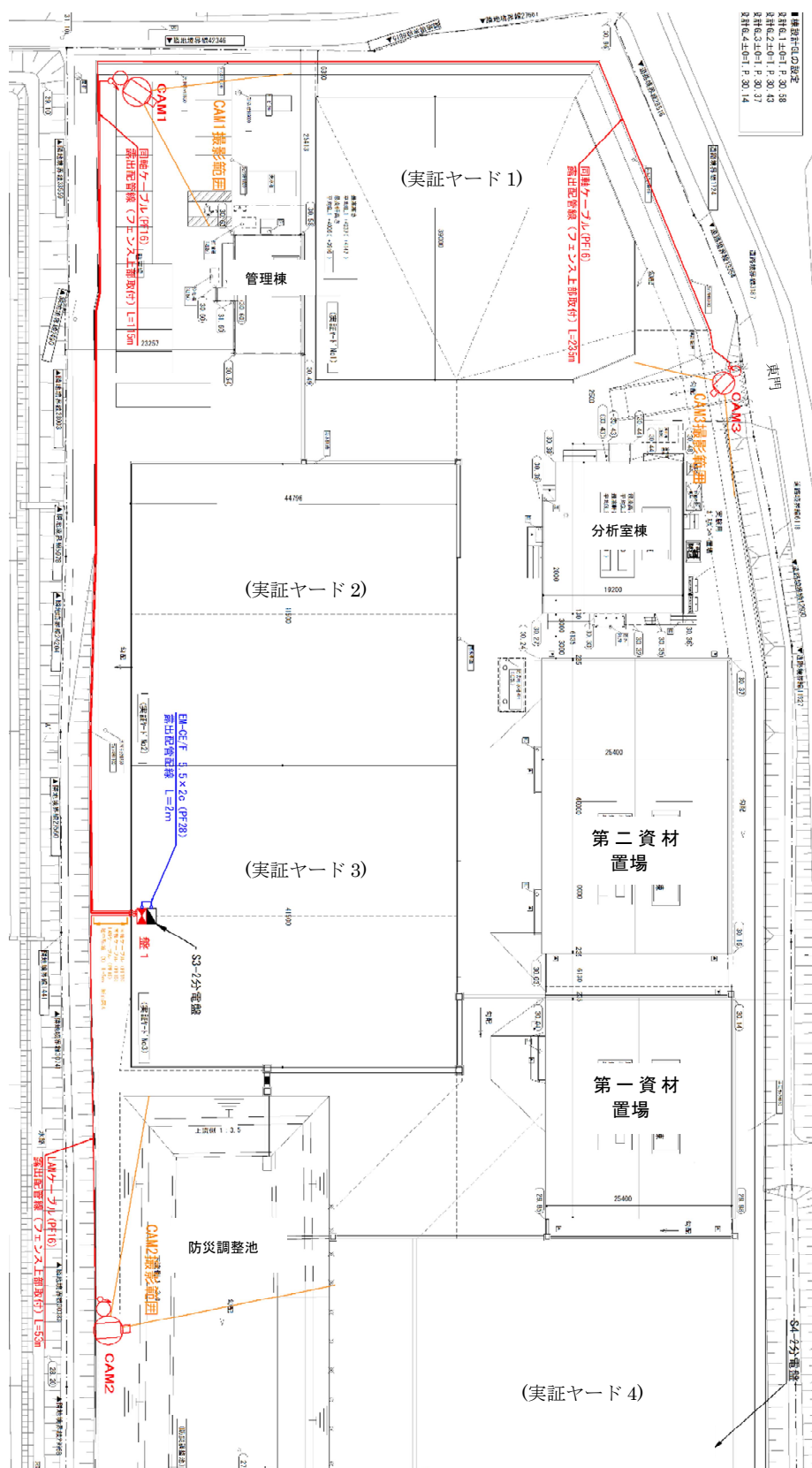
別紙1-1 設置配置図（技術実証フィールド 屋外 CAM1、2、3）
