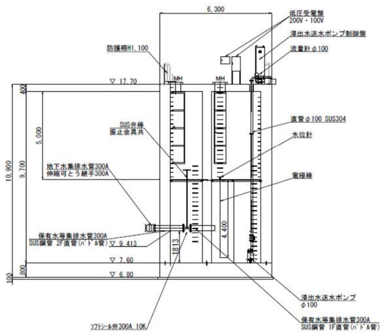
浸出水集水ピット断面図(B-B)
