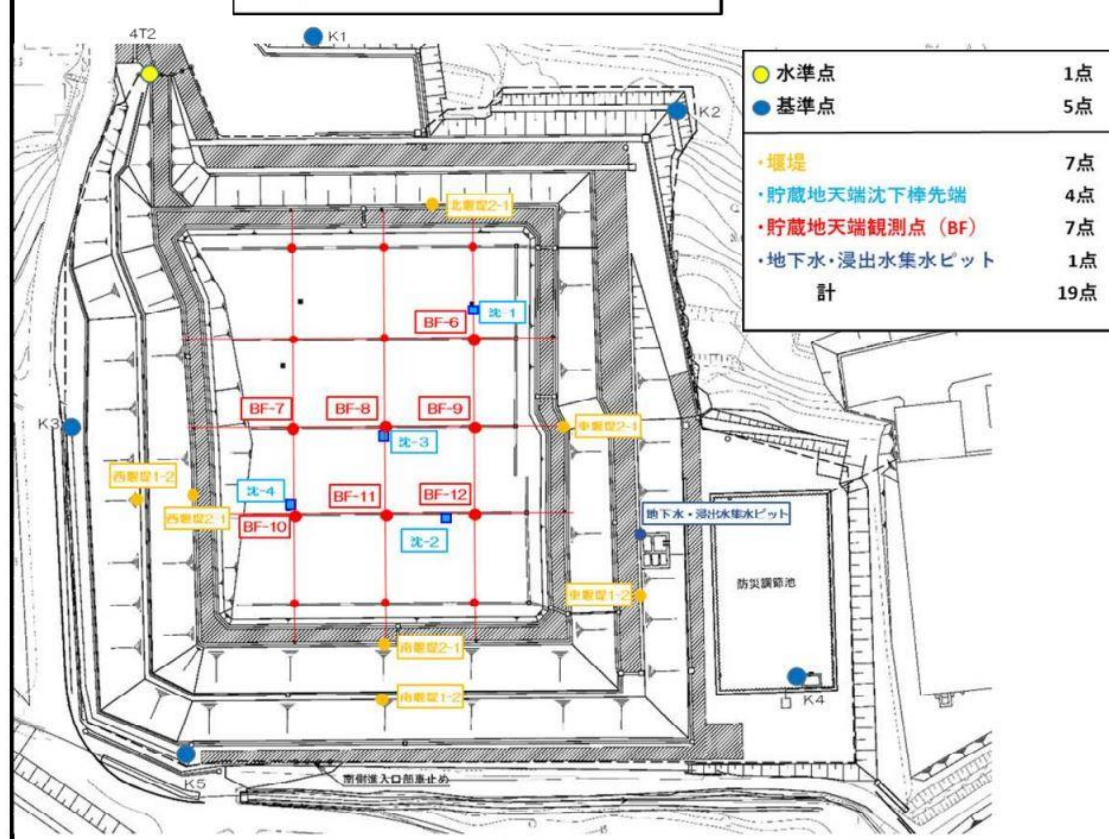
双葉①工区東側 土壌貯蔵施設 計測点位置
