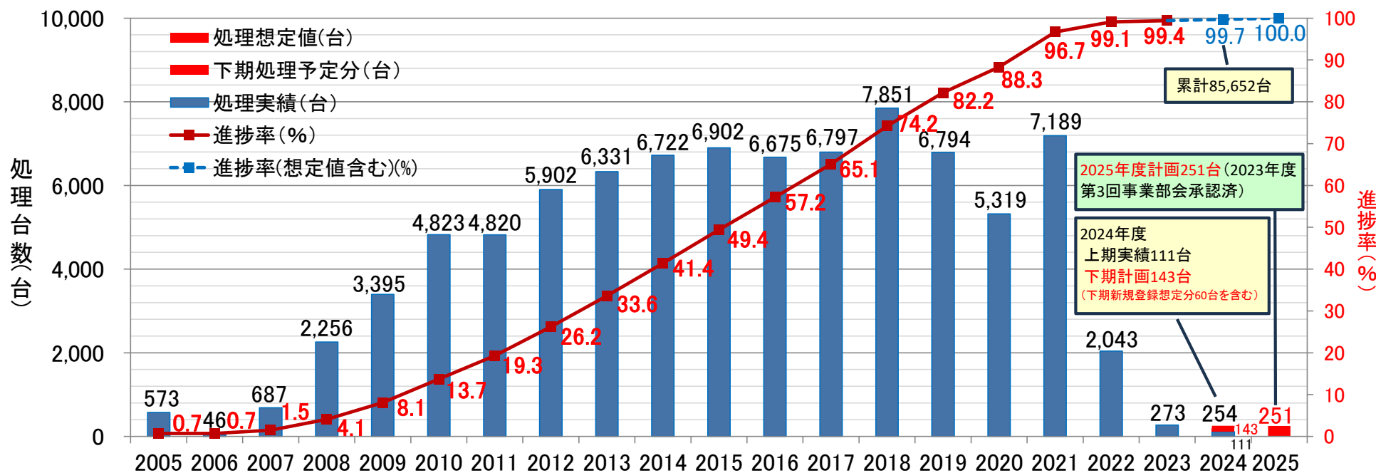
図5 コンデンサーの操業開始時からの処理実績と今後の処理計画
